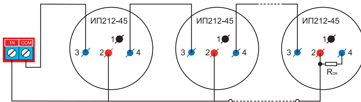
Рисунок 3. Схема подключения ИП212-45 к пожарному входу NV 216 только с оконечным резистором
