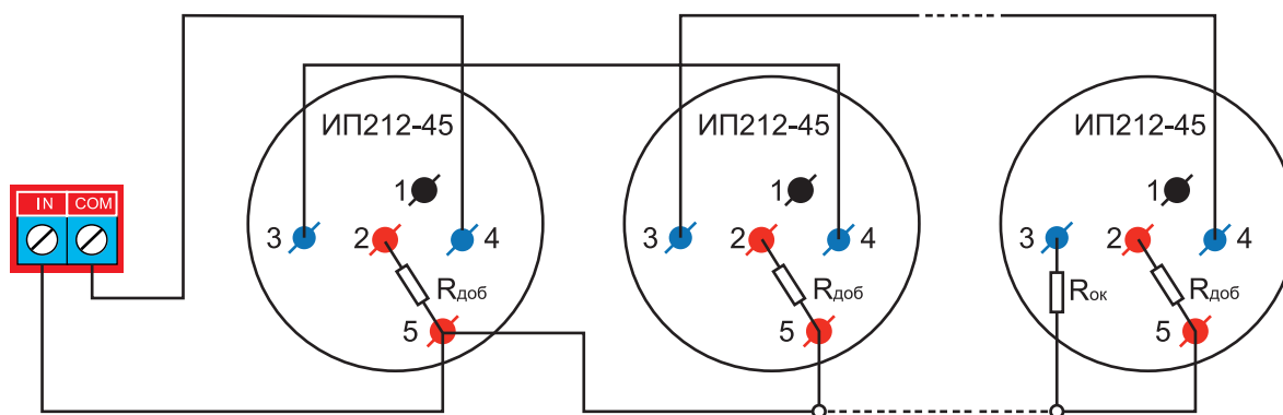
Рисунок 2. Схема подключения ИП212-45 к пожарному входу NV 216 с добавочными и с оконечным резисторами
