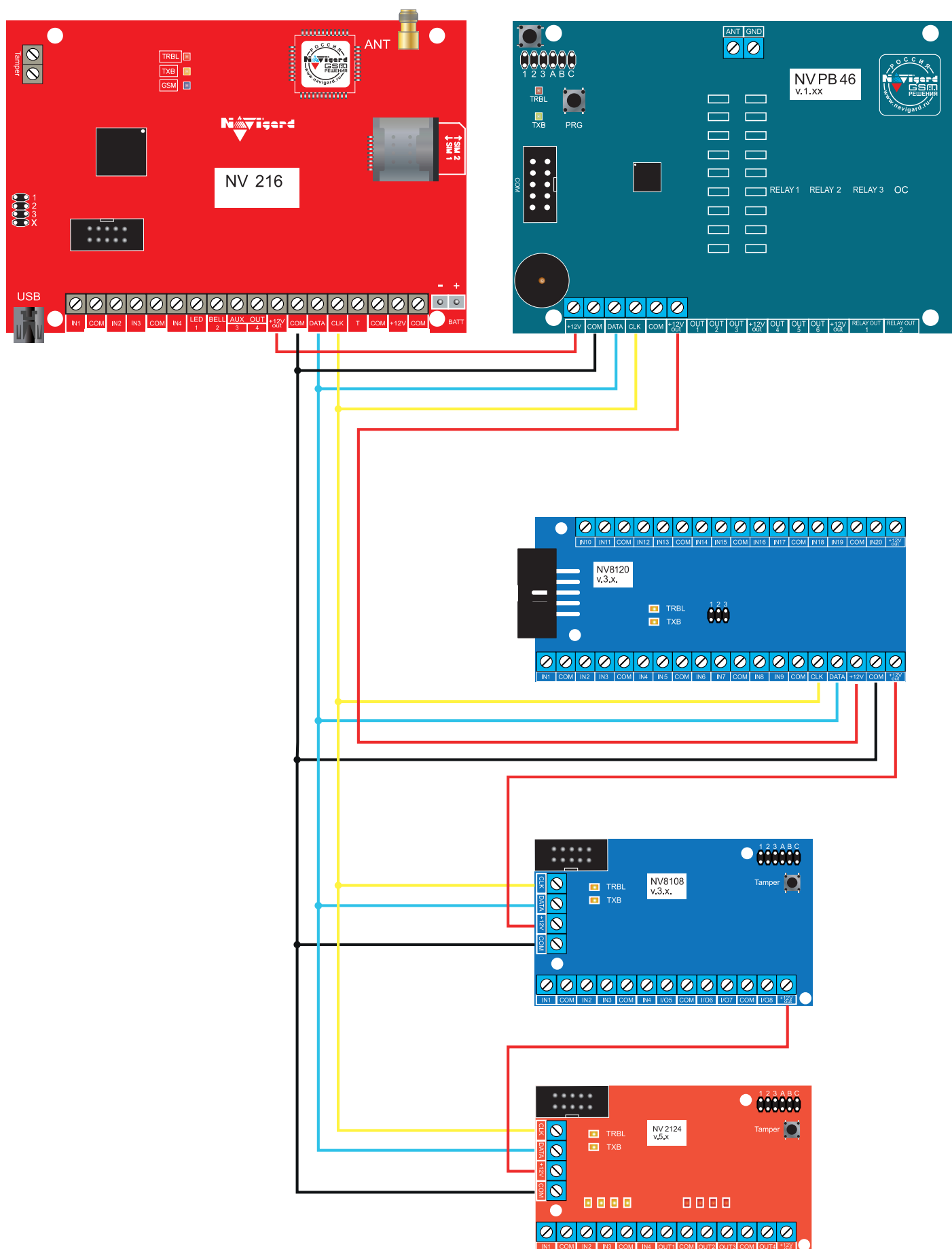
Рисунок 19. Подключение нескольких расширителей по системной шине
