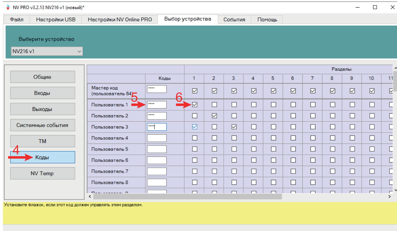
Рисунок 17. Вкладка Коды в NV Pro
