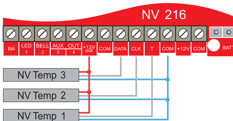
Рисунок 4. Подключение датчиков температуры NV TEMP
